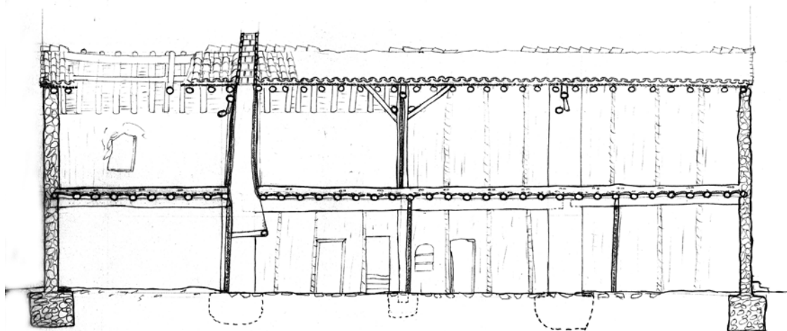
SECCIÓN LONGITUDINAL
